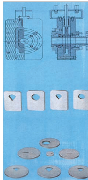
Drehschieberventil mit keramischen Schieberplatten
