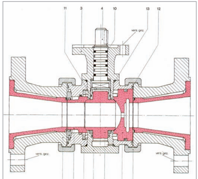
Schnittzeichnung durch einen Kugelhahn
