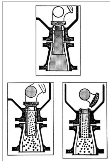
Einfluß der Abströmhülse auf die Strömung beim Öffnen des Drehkegels
