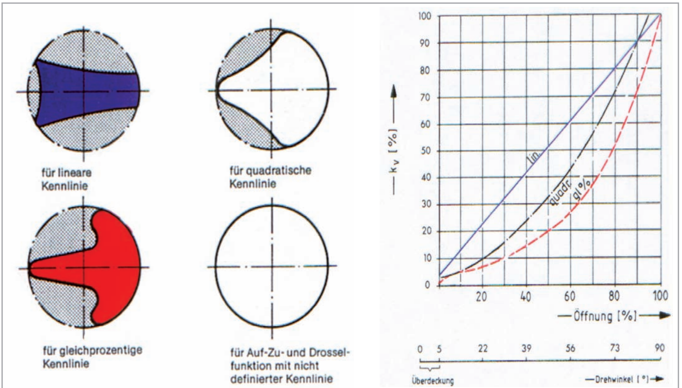
Regelprofile der Regelscheiben für lineare, quadratische und gleichprozentige Kennlinien
