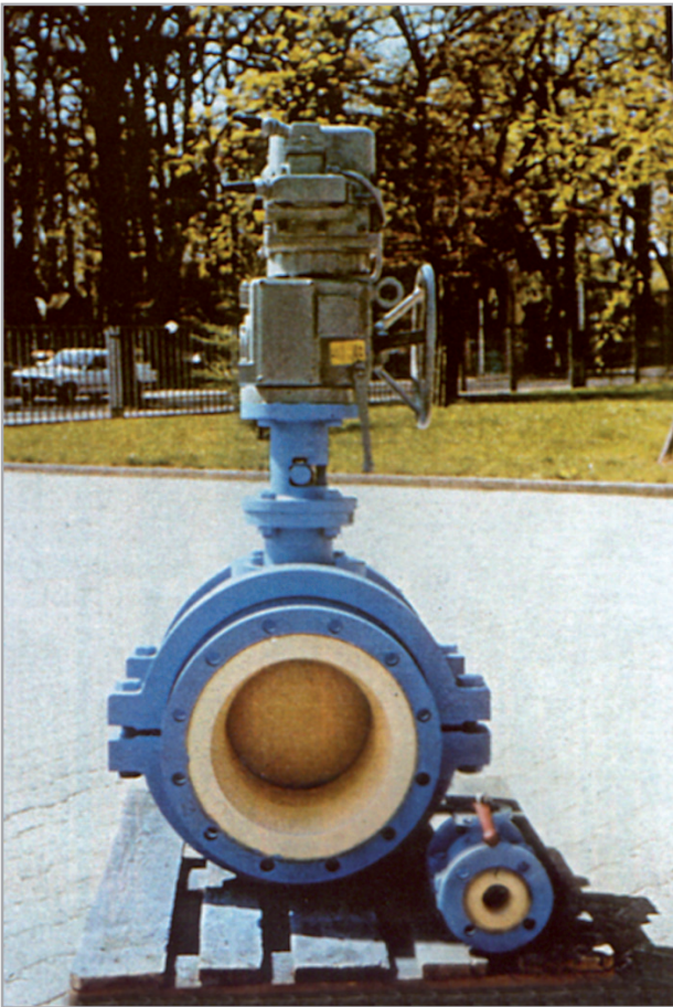
Kugelhahn DN350 und DN50 aus Aluminiumoxid
