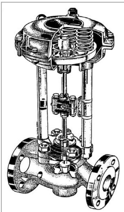
Regelventil/Hubventil
