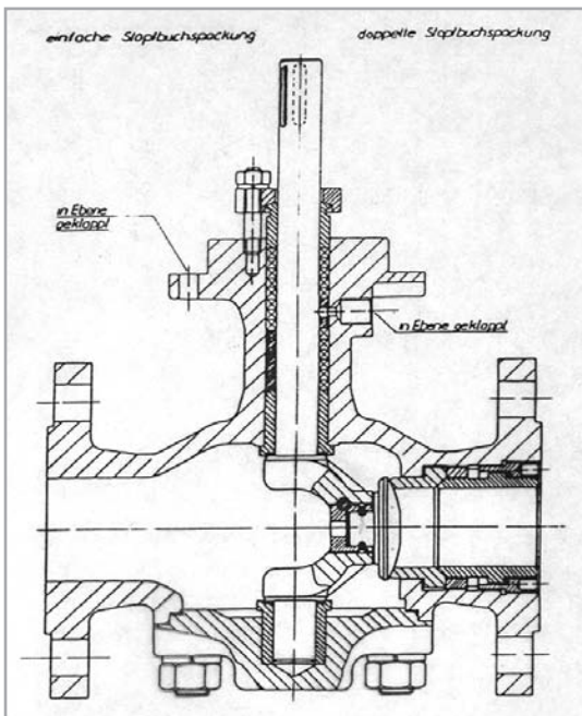
Drehkegelventil-Sc hnttzeichnung
