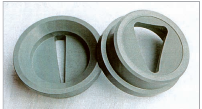
Regelscheiben aus Siliziumnitrid
